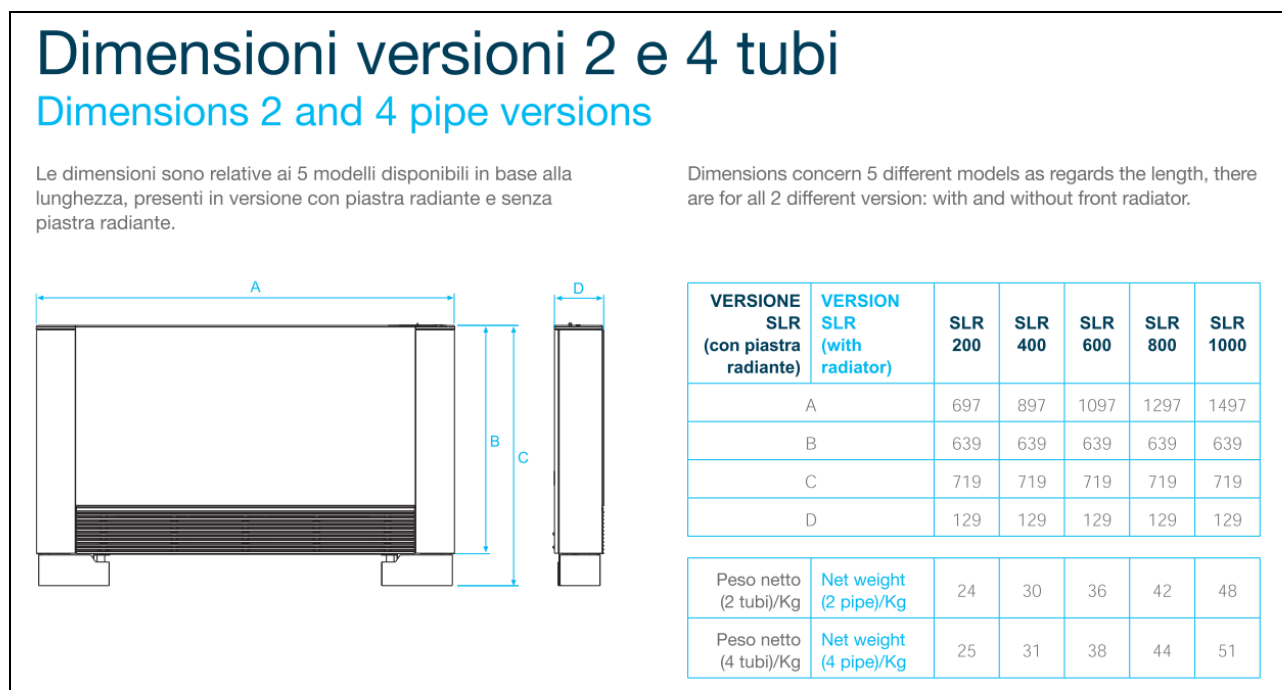
Figura 1 - Dimensionali
